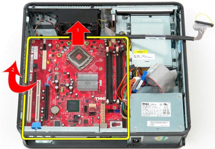
51. החלק את לוח המערכת לכיוון גב המחשב והרם אותו מחוץ מהמחשב.
