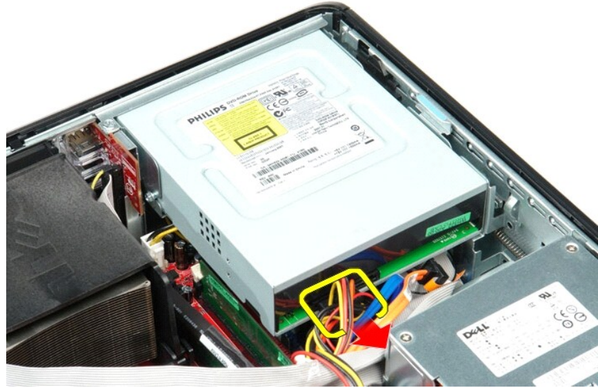
4. משוך את תפס שחרור הכונן והזז את הכונן כלפי גב המחשב.
