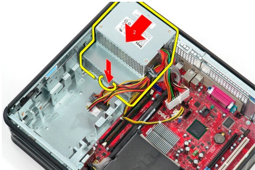
9. הרם את ספק הכוח והוצא אותו מהמחשב.
